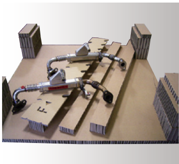
緩衝材
